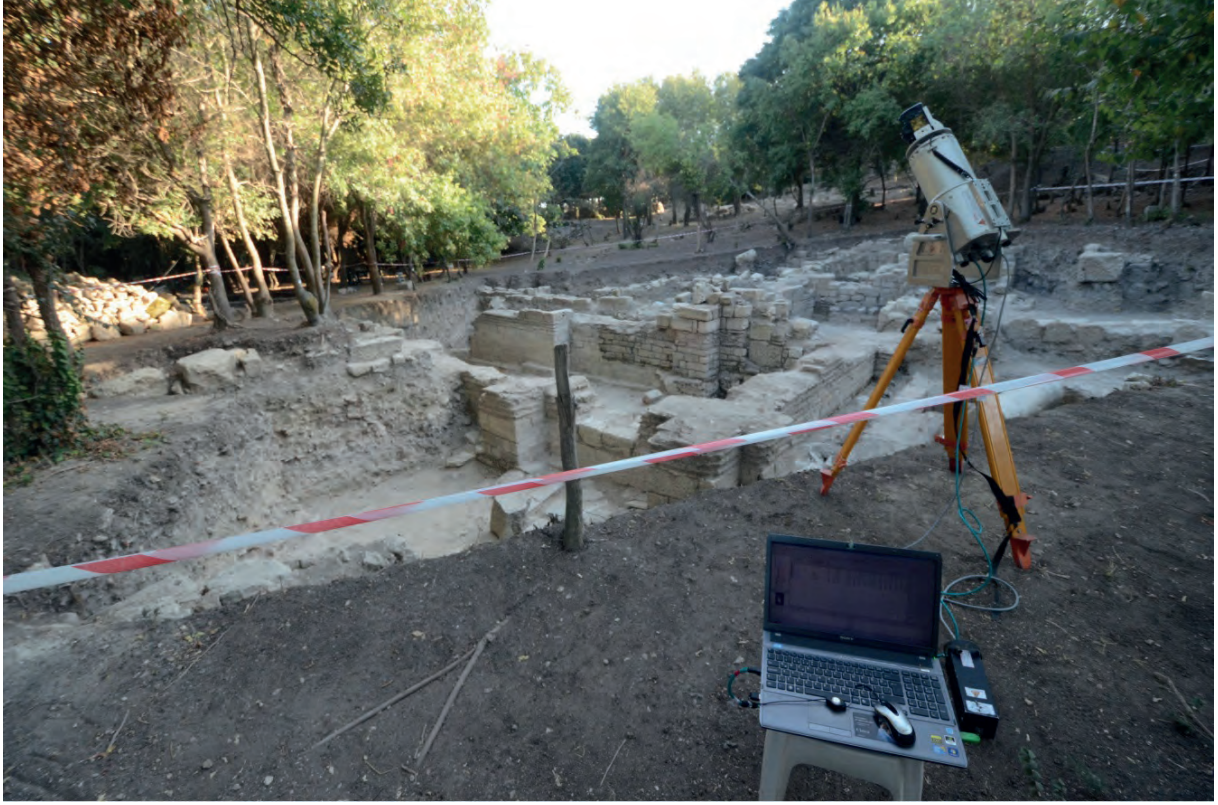
Res. 25: Sütunlu yapıda yürütülen 3B ölçüm çalışmaları Fig. 25: 3D scanning carried out in the building with column
